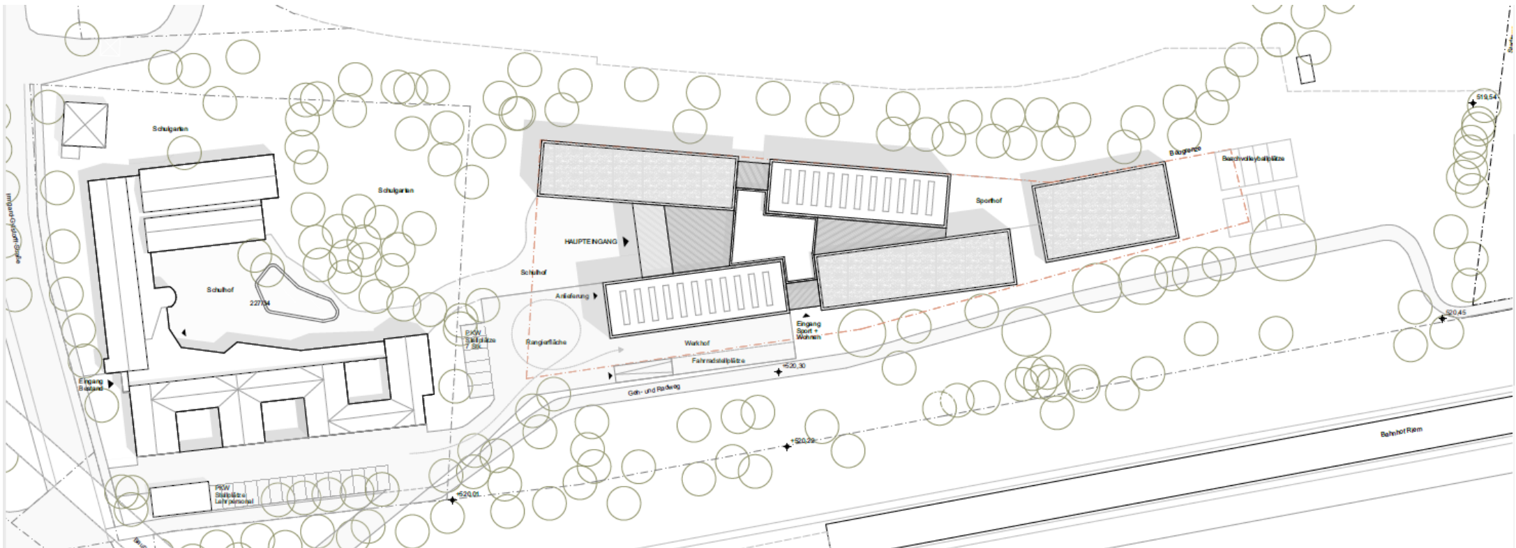
Lageplan
