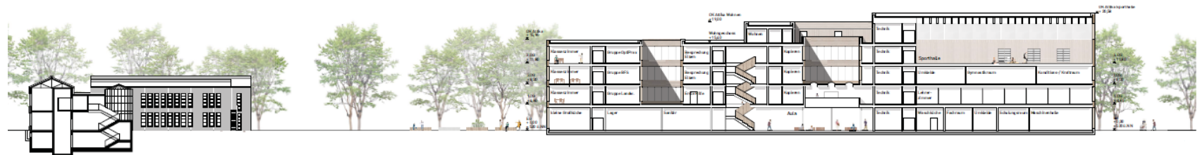
Systemschnitt
