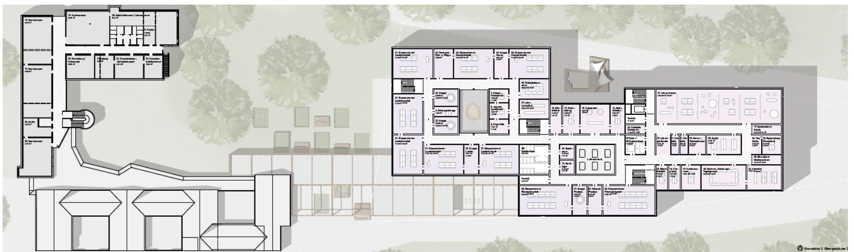
Grundriss 1. Obergeschoss
