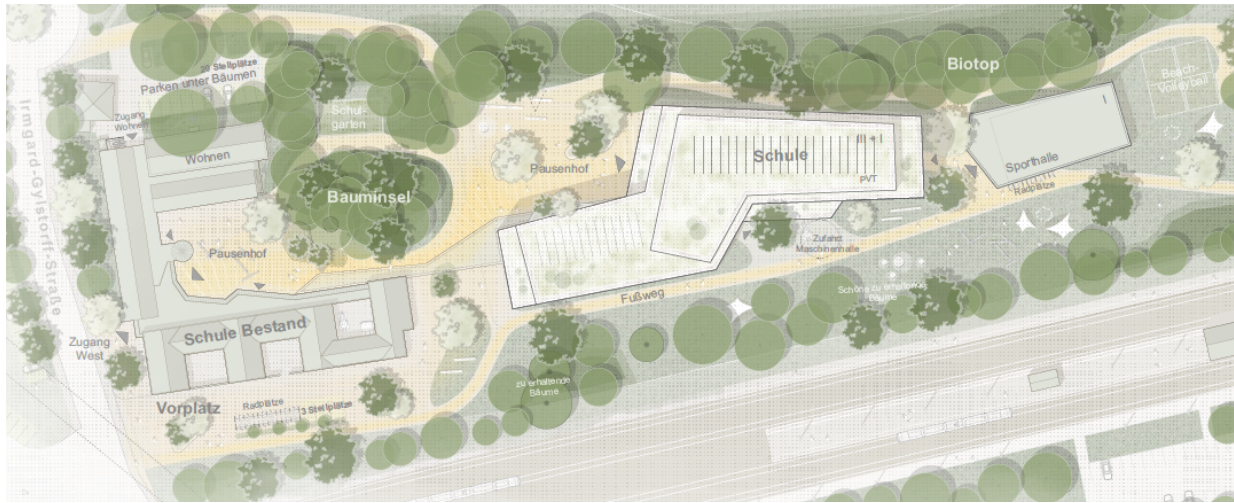
Lageplan
